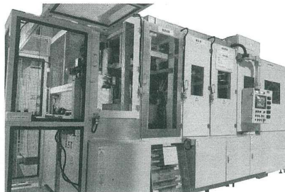
全自動磁粉探傷装置
